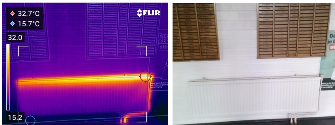
Foto's: waterzijdig ingeregelde radiator gezien door de warmtecamera (links) en de gewone camera (rechts).
